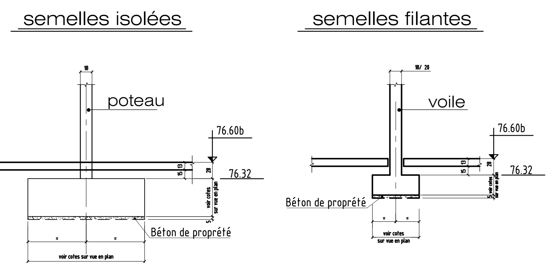
principe de fondations Coupe type
