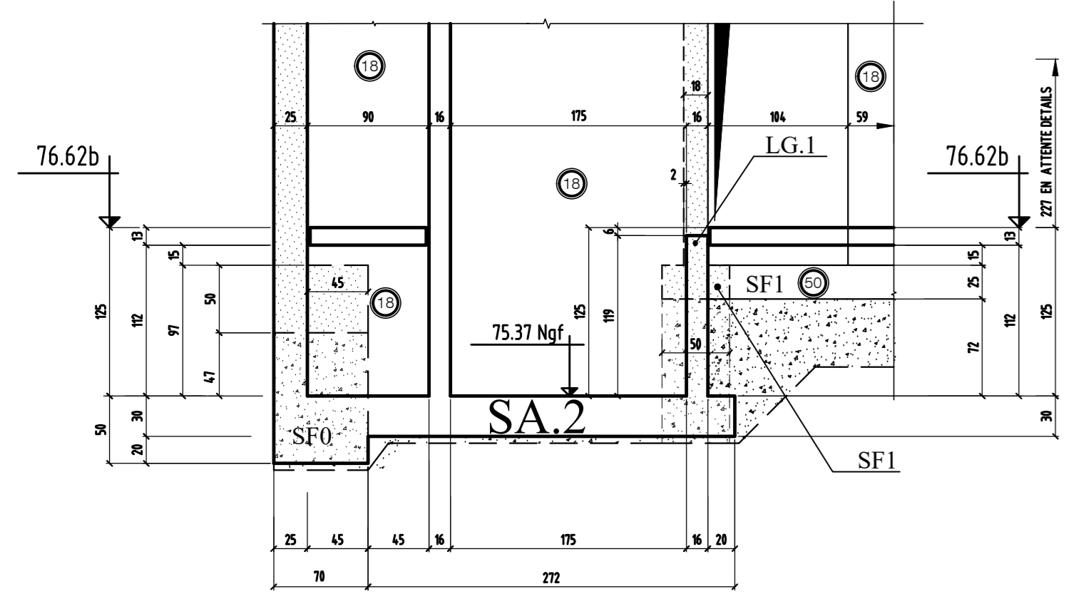
Coupe 2-2 en attente détails ASC
