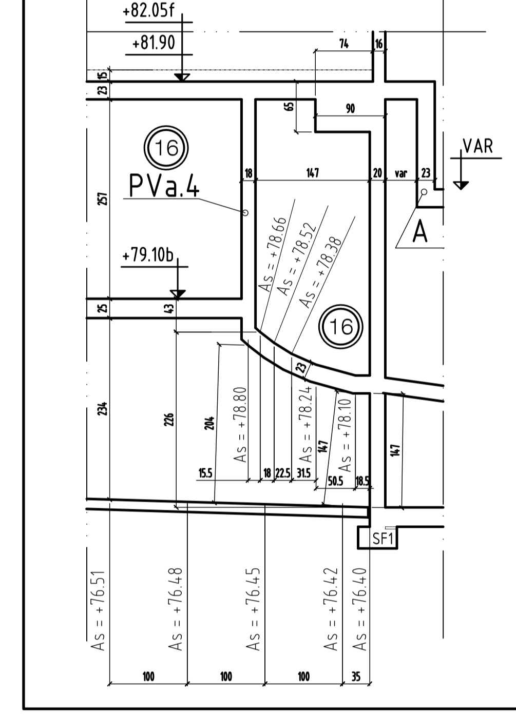
COUPE 4-4
