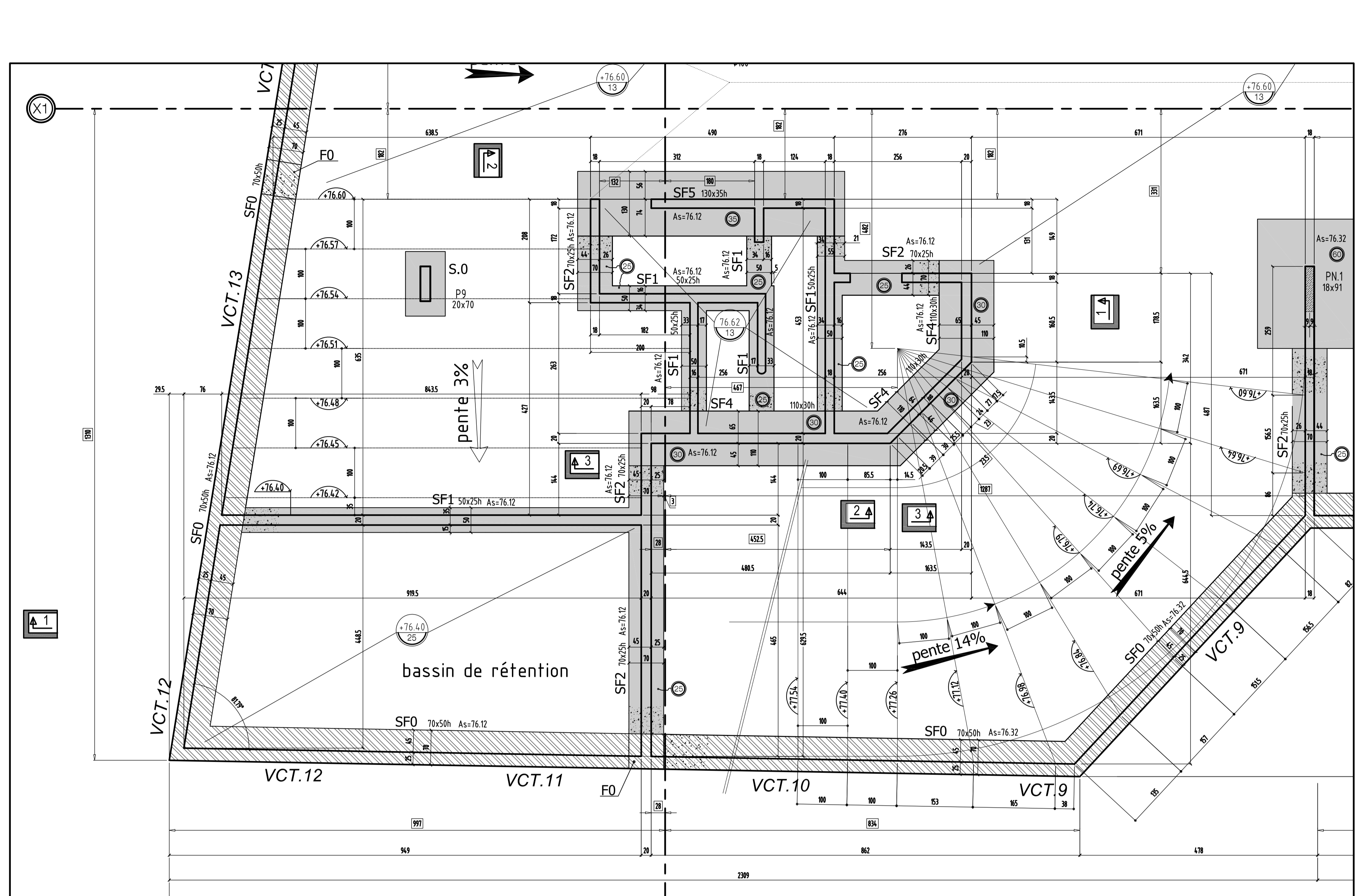
VUE EN PLAN -FONDATIONS
