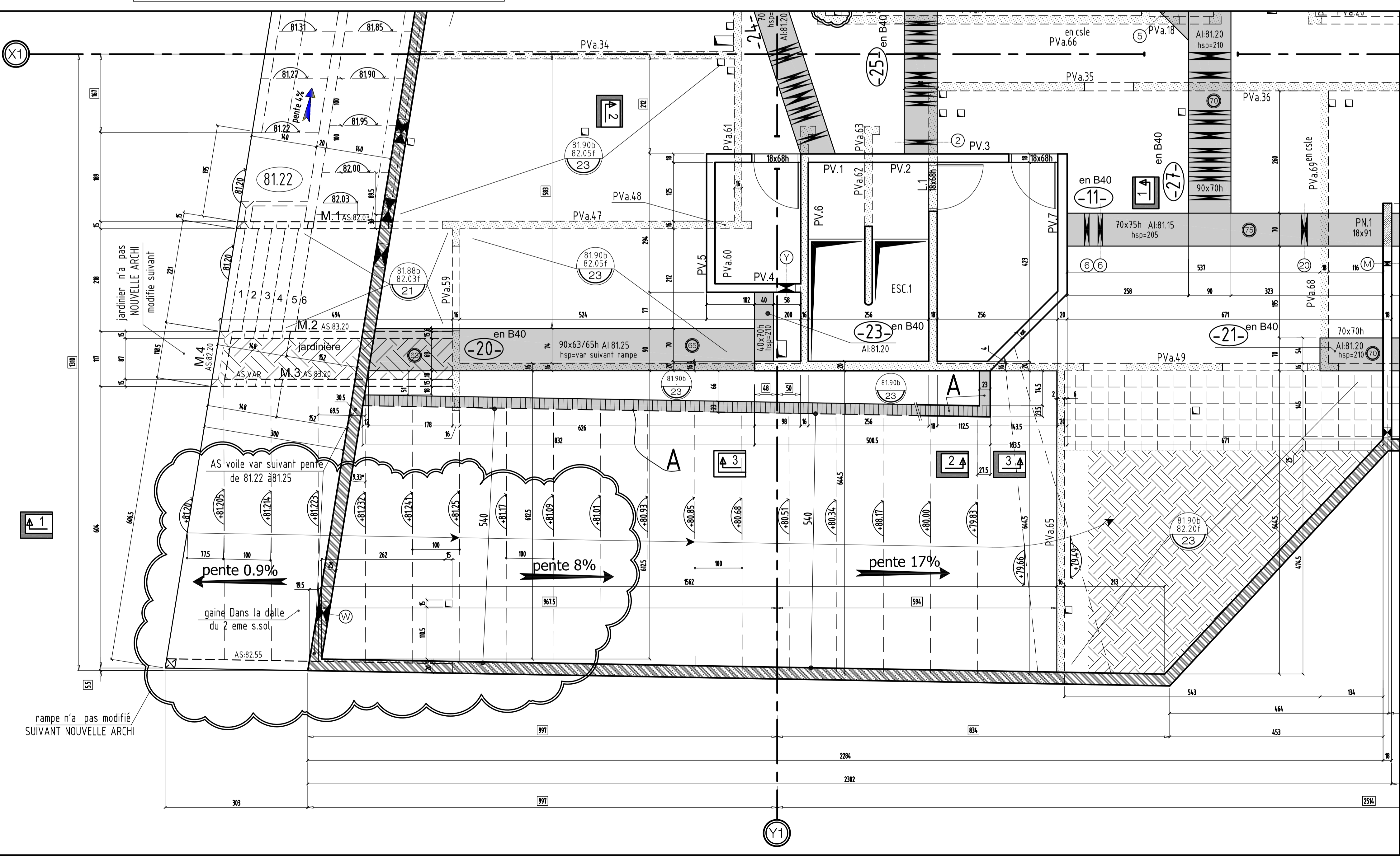
VUE EN PLAN -PH SS-1
