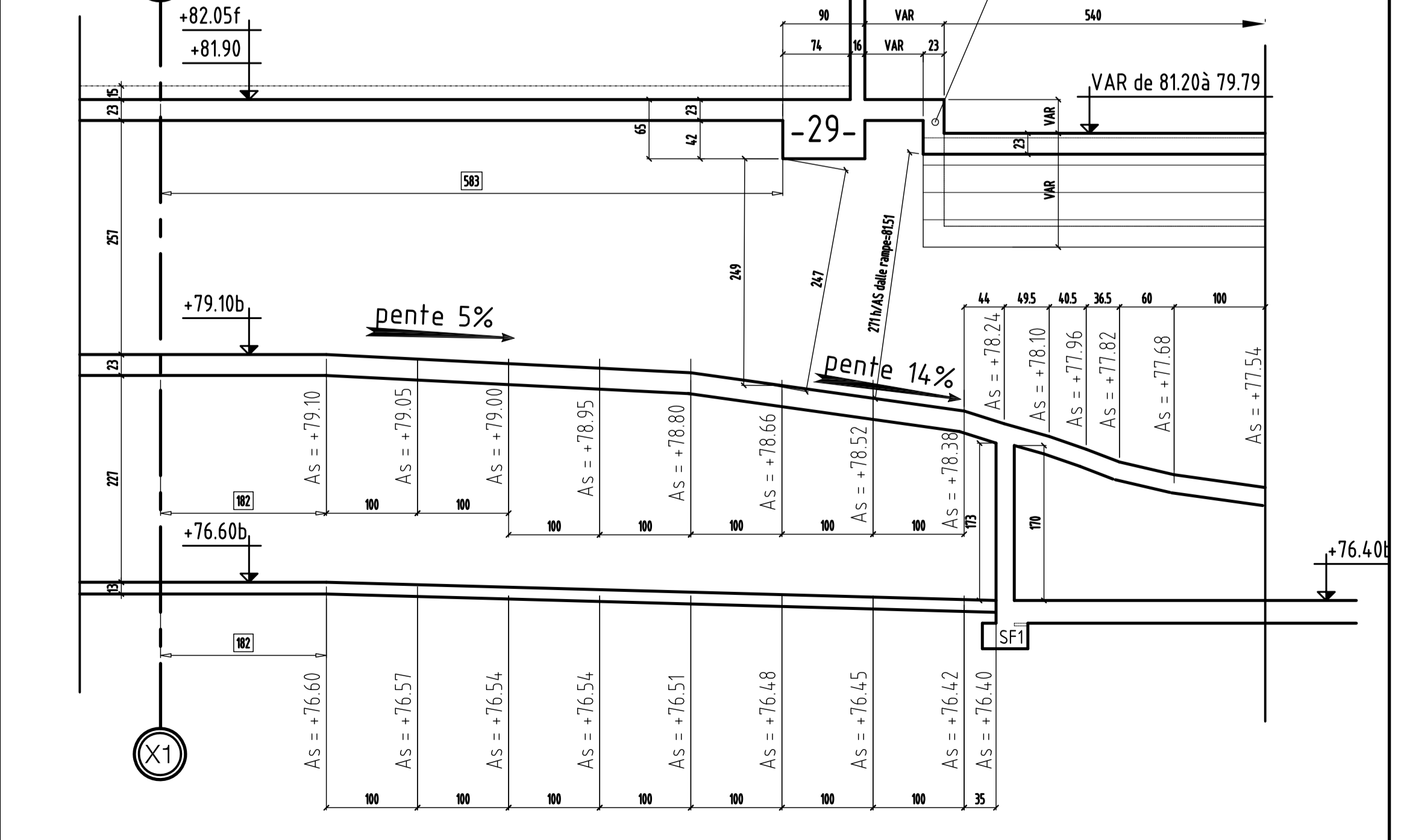
COUPE 2-2
