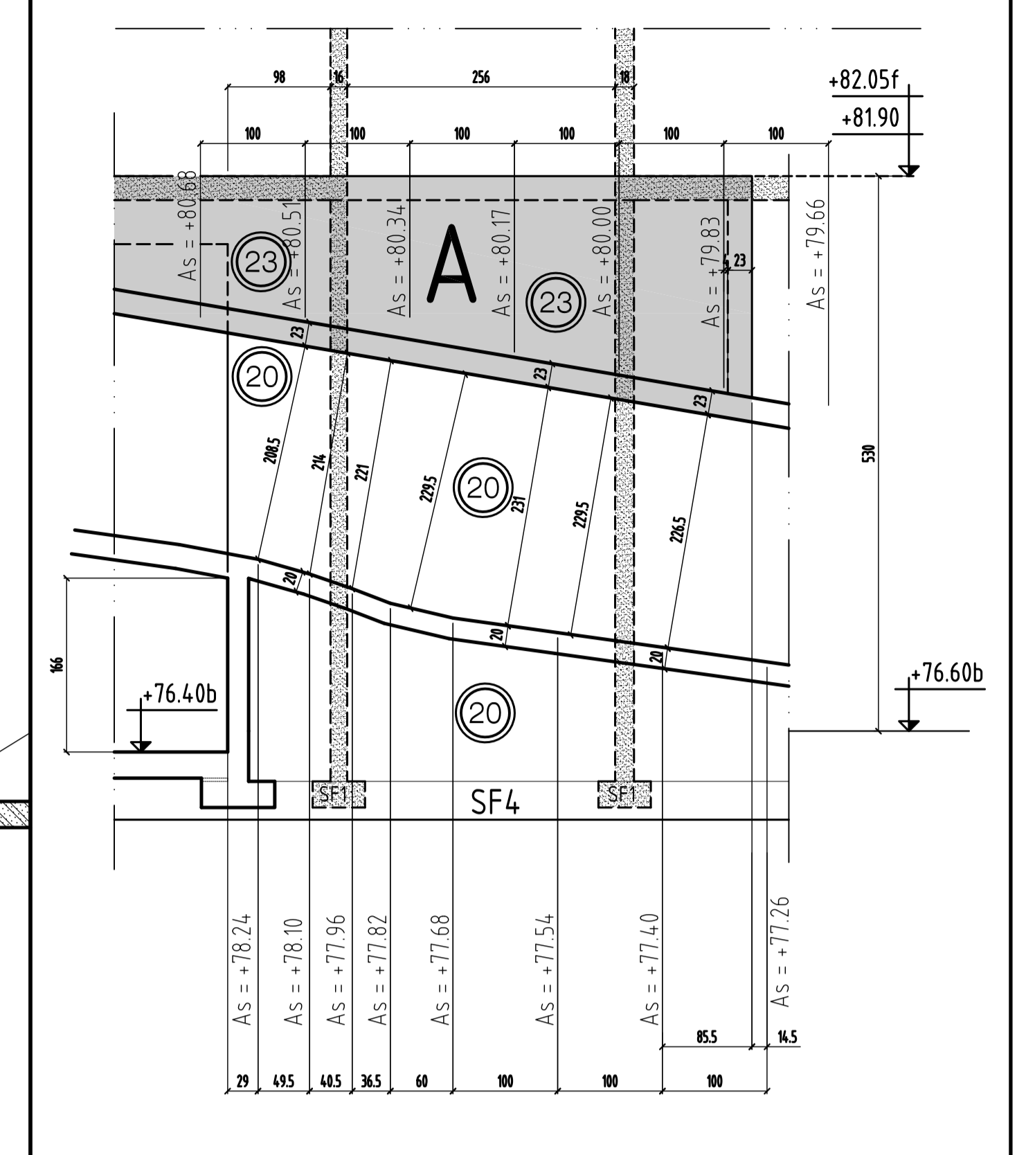
COUPE 4-4
