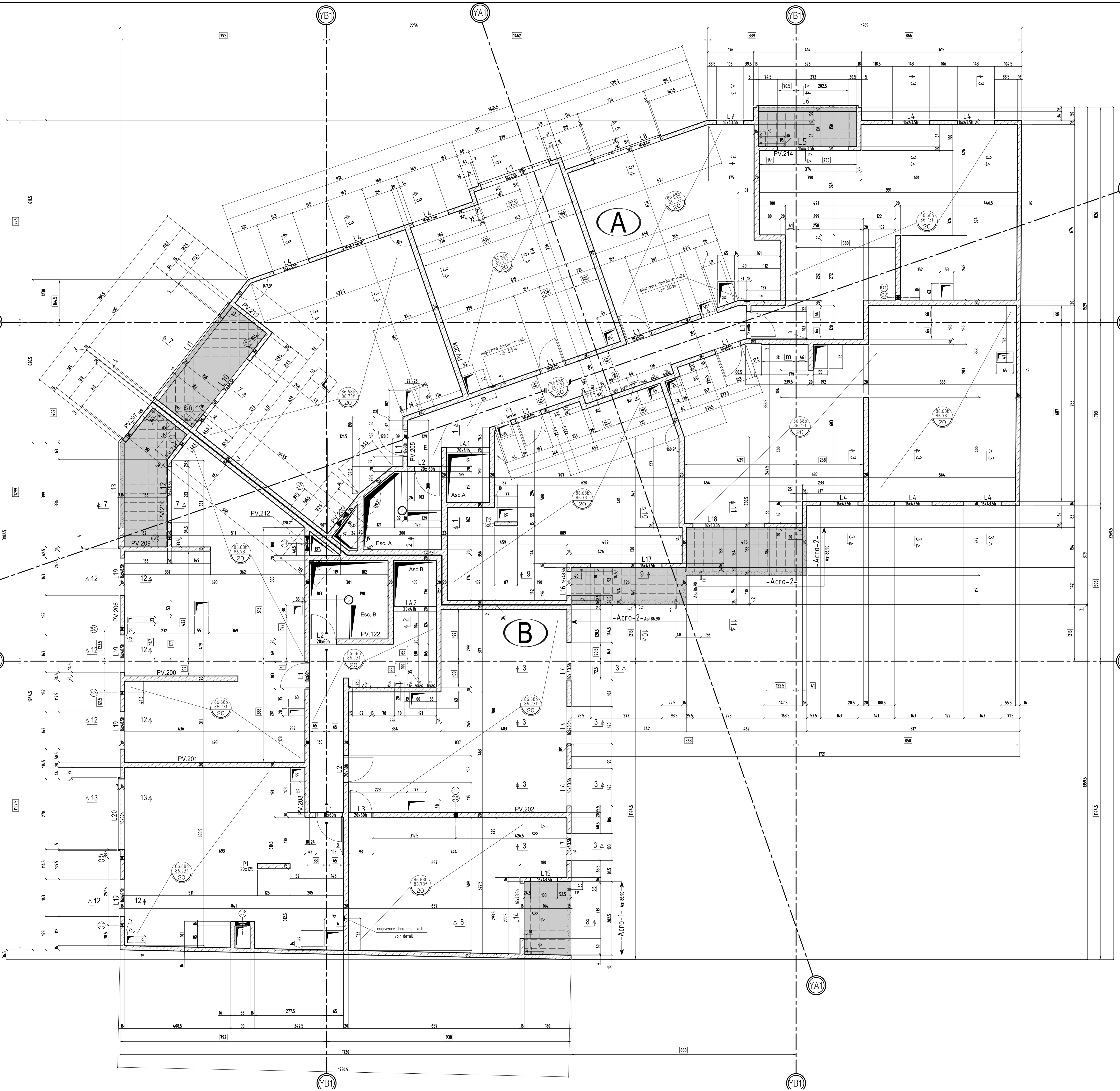
VOIR PLAN N° : C.11 - Coupes et détails
