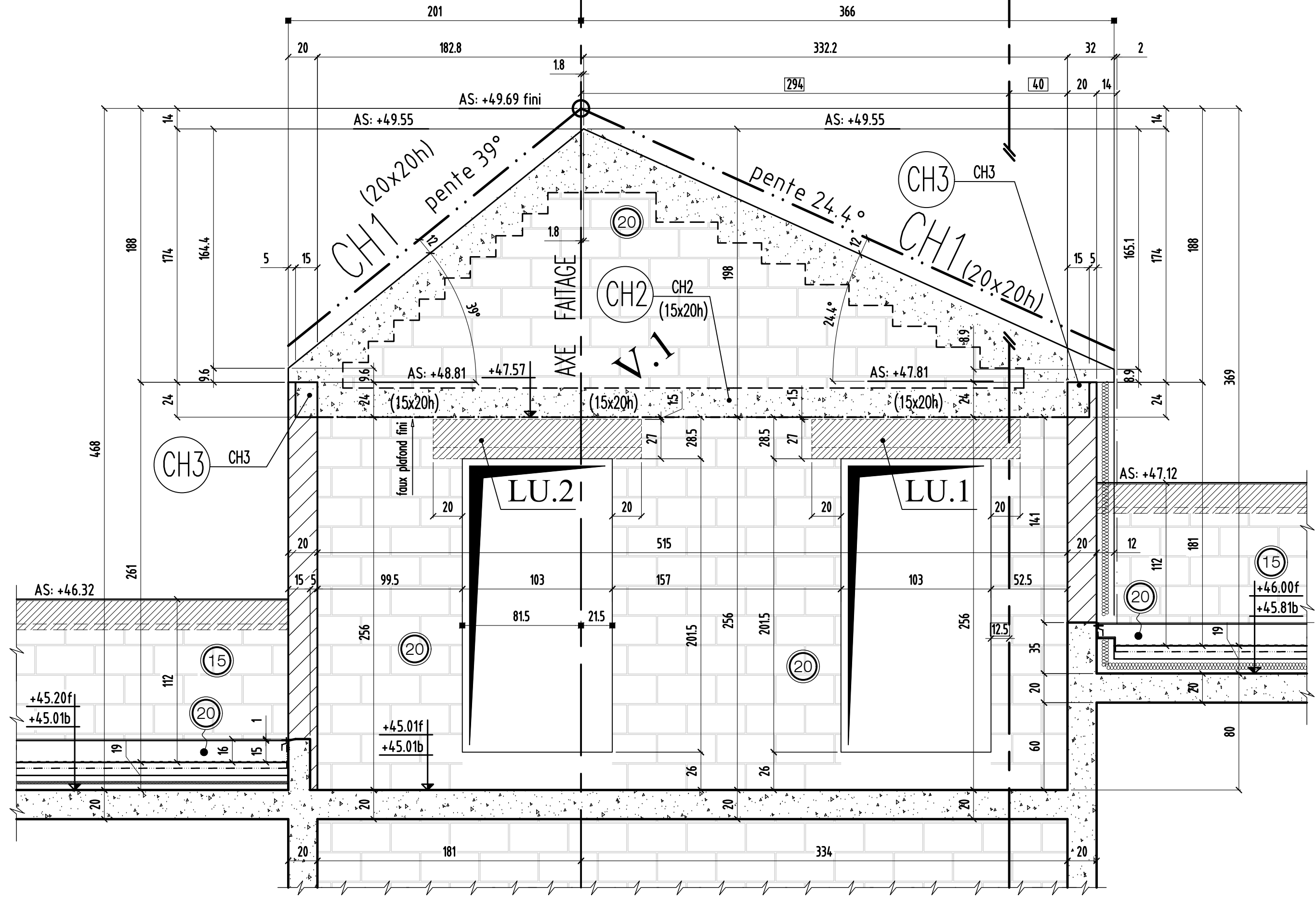
coupe 2-2
