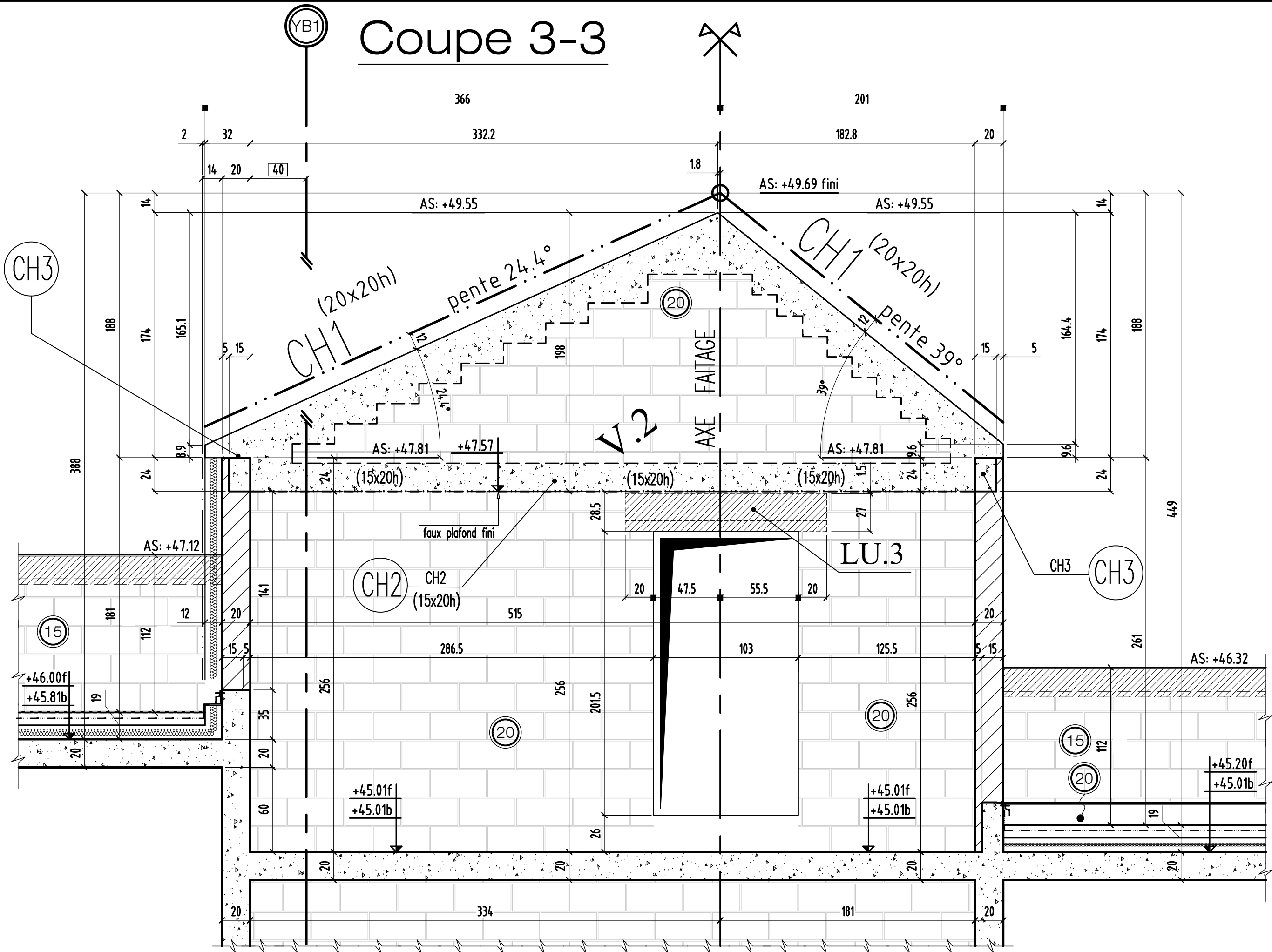
Coupe 3-3
