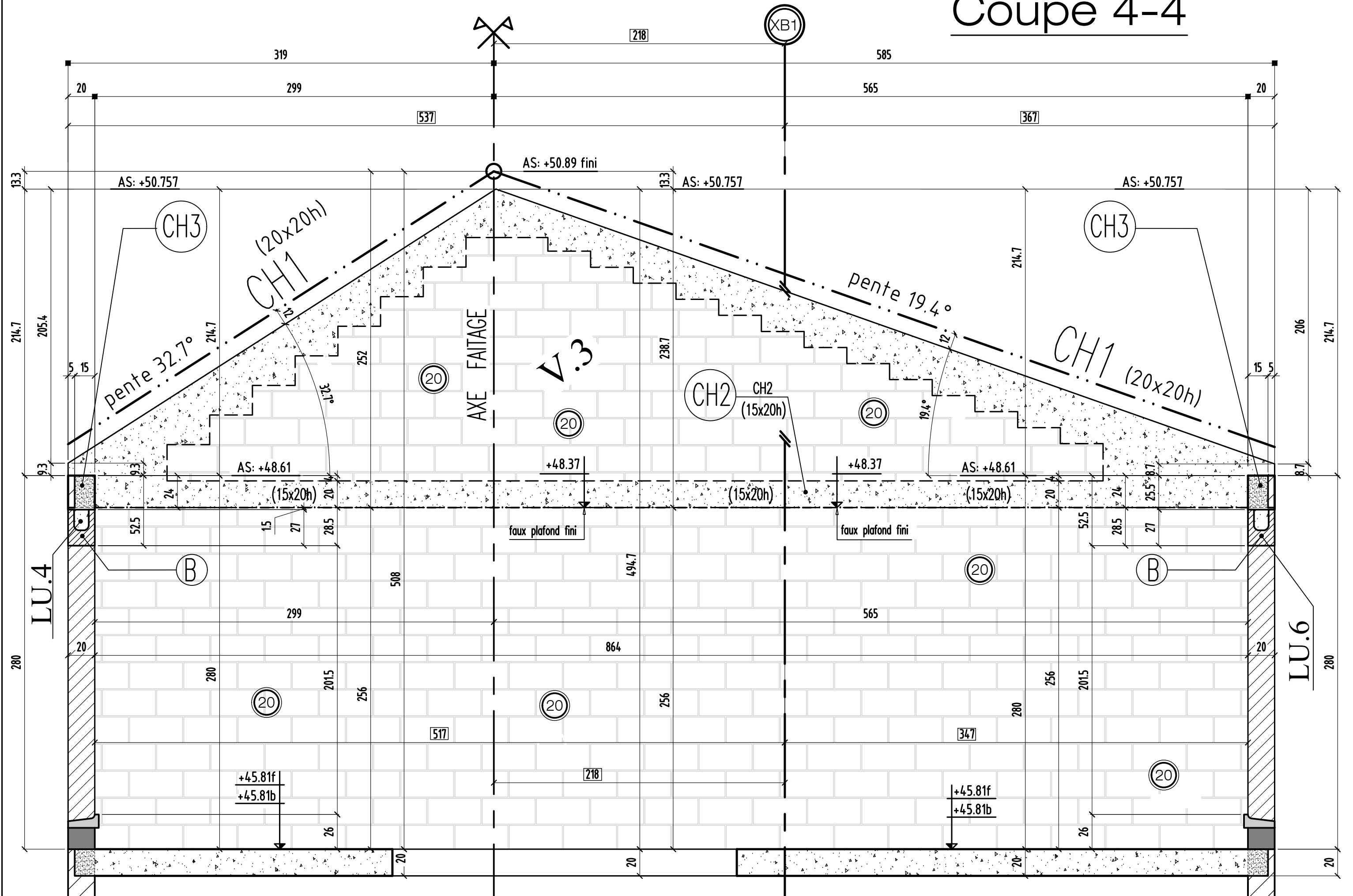
Coupe 4-4
