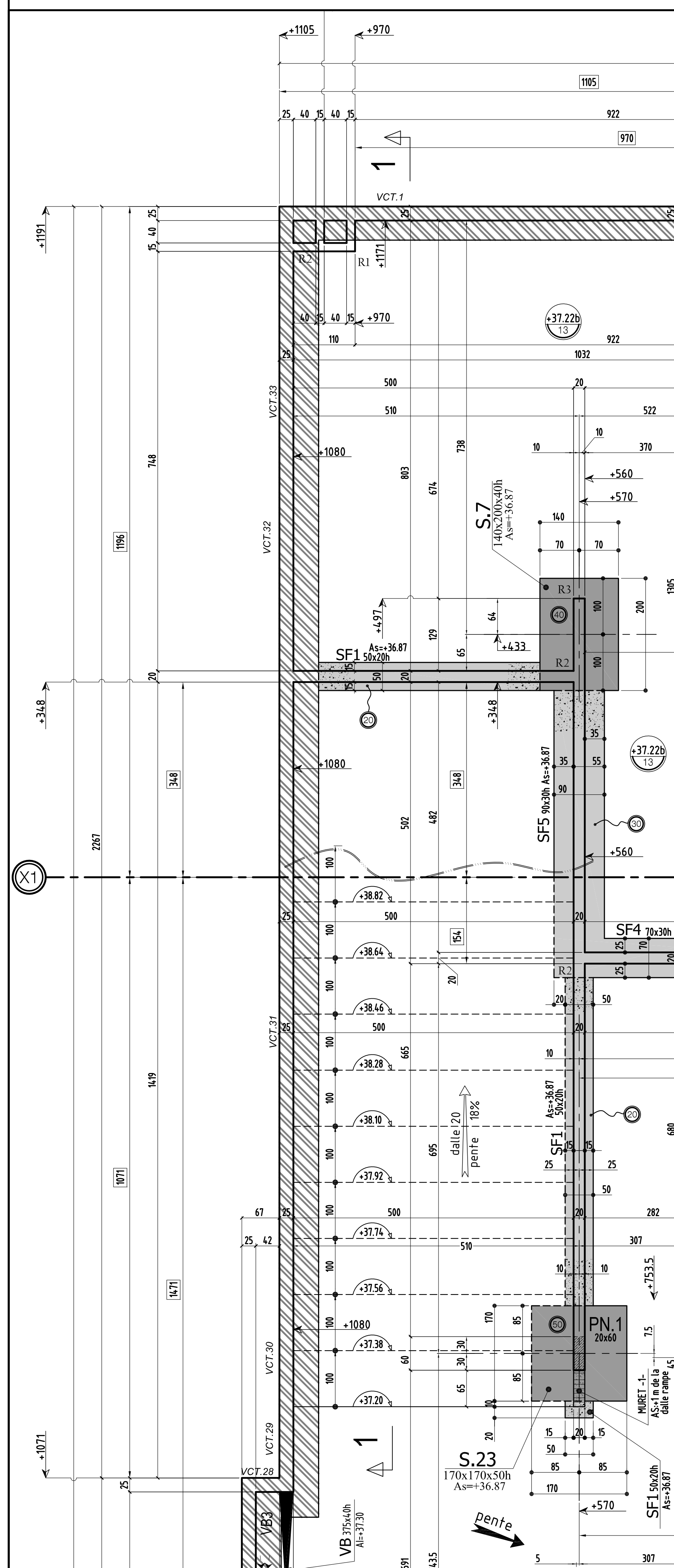
VUE EN PLAN -Fondation
