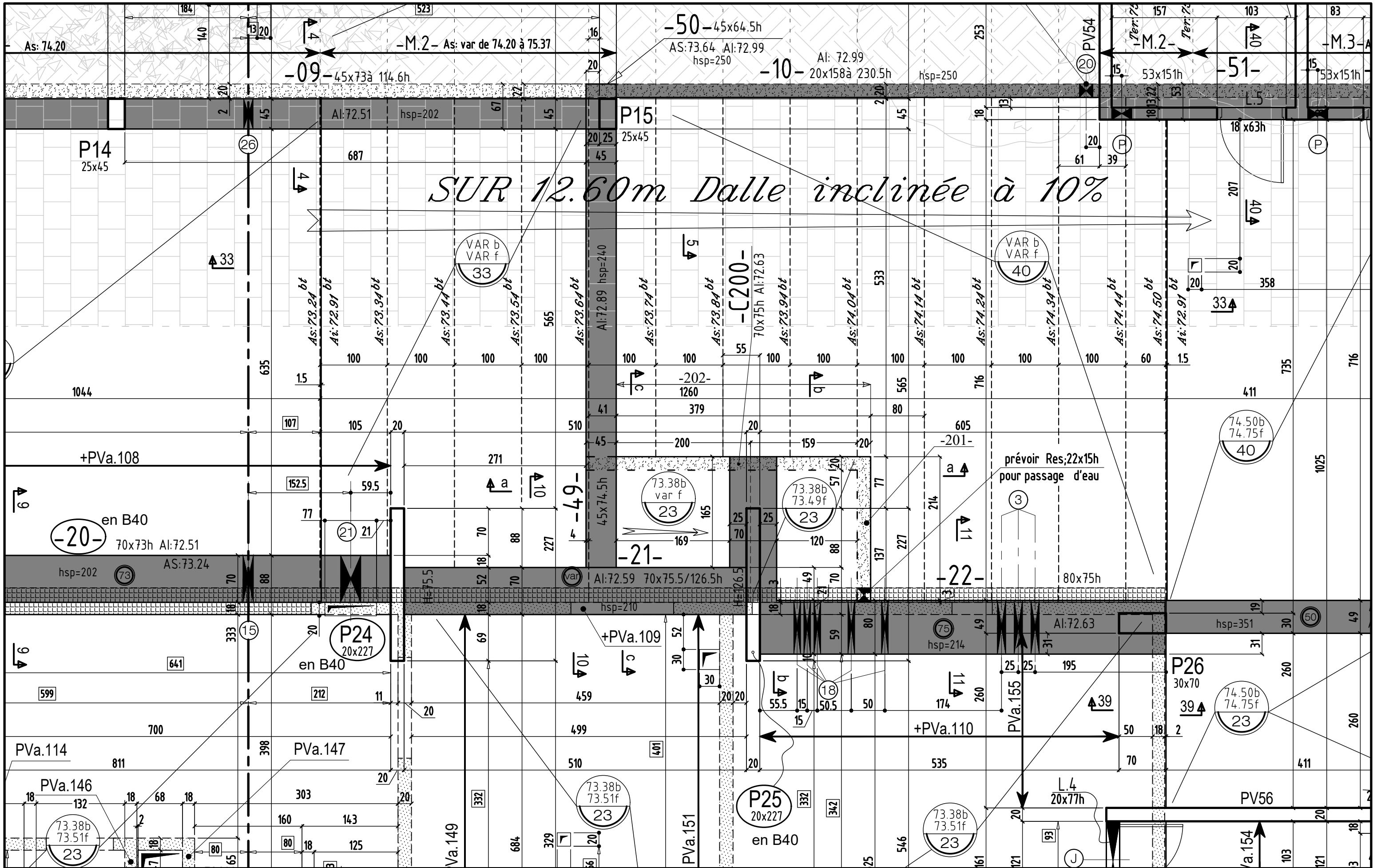
VUE EN PLAN (Vue de dessous) - COFFRAGE
