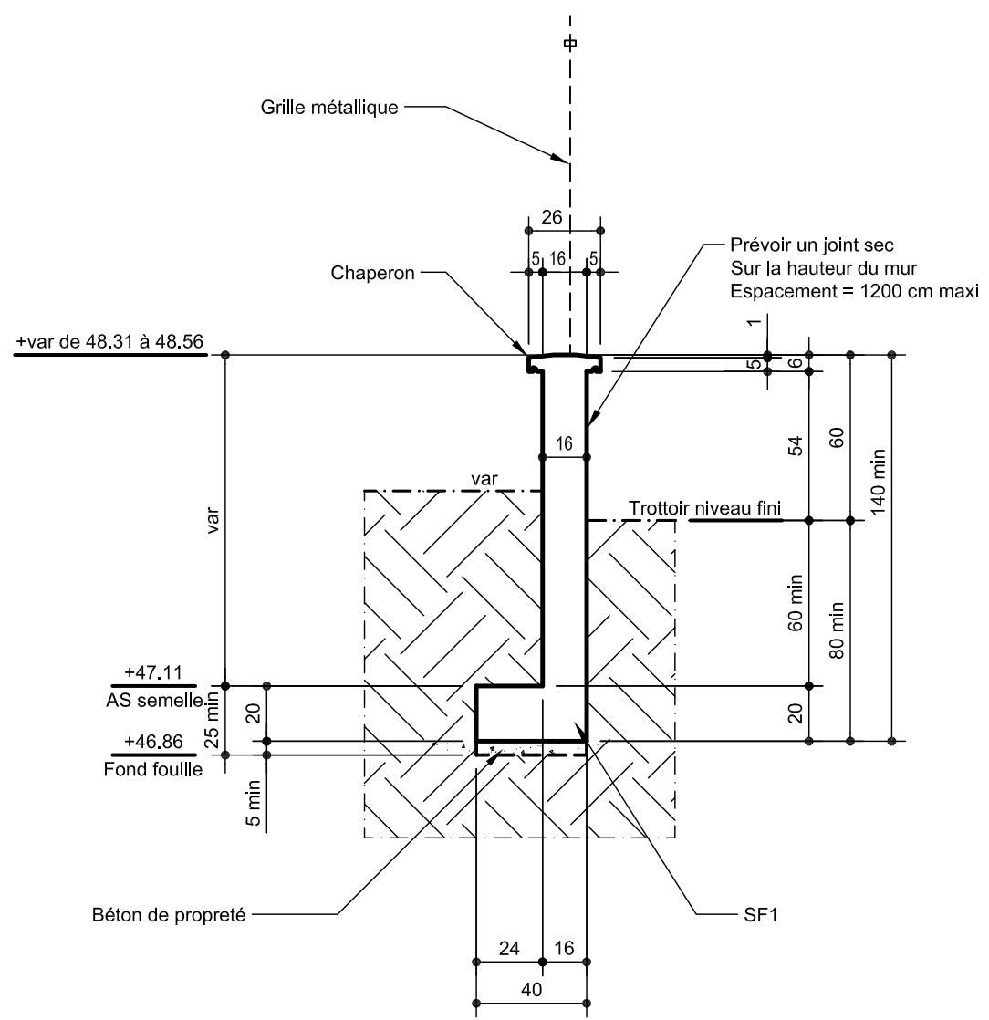
COUPE 3-3 M.3
