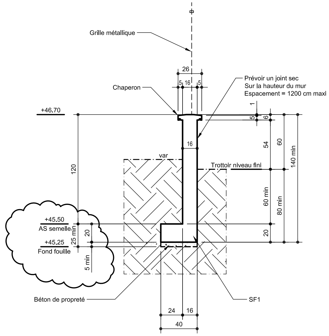
COUPE 1-1 M.1
